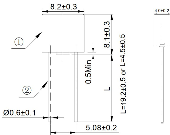
6-1 工程圖 ( 單位 : mm ) / Outline Drawing and Dimensions (Unit: mm)
