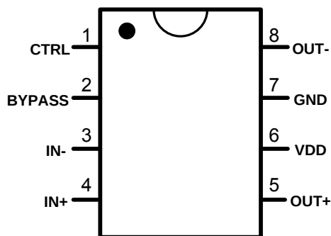
顶视图
