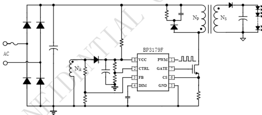
图 1 BP3179F PWM 调光典型应用图
