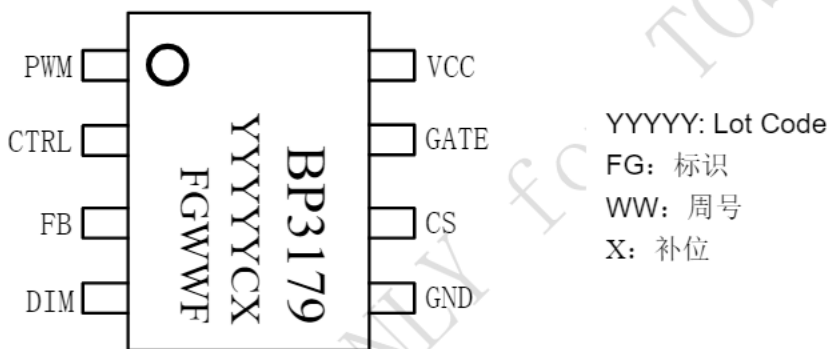
图 3 管脚封装图
